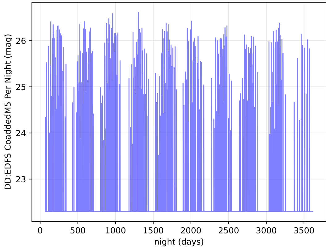
ddf_acor_sf10_lsf30_lsr50_v3.4_10yrs g band: DD:EDFS CoaddedM5 Per Night
