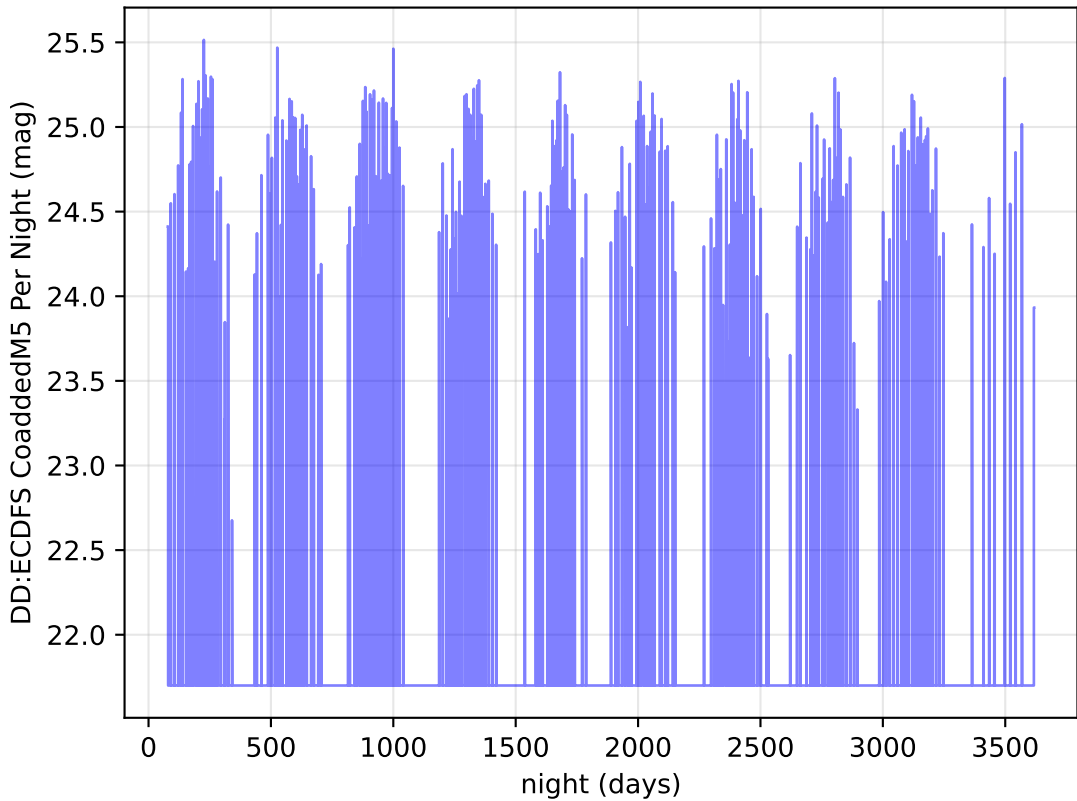
ddf_acor_sf10_lsf30_lsr50_v3.4_10yrs z band: DD:ECDFS CoaddedM5 Per Night
