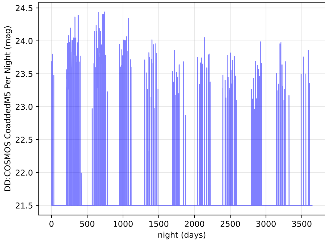
ddf_acor_sf10_lsf30_lsr50_v3.4_10yrs y band: DD:COSMOS CoaddedM5 Per Night
