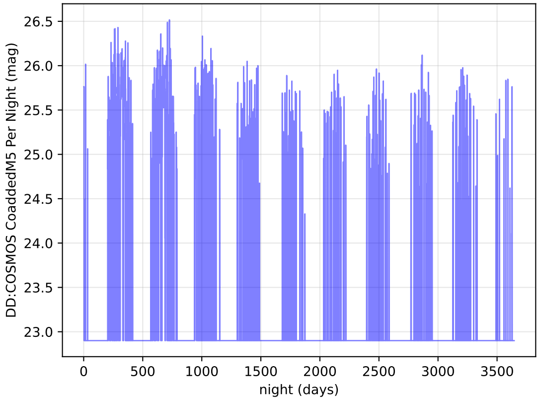
ddf_acor_sf10_lsf30_lsr50_v3.4_10yrs r band: DD:COSMOS CoaddedM5 Per Night
