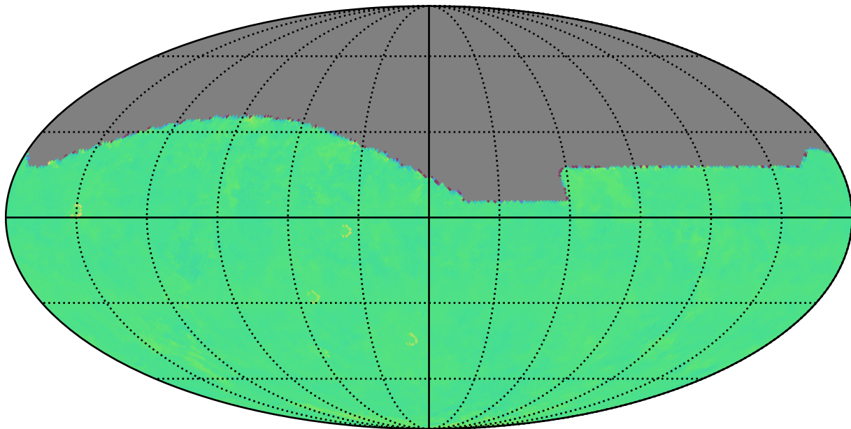
ddf_acor_sf10_lsf30_lsr20_v3.4_10yrs i: Kuiper rotTelPos
