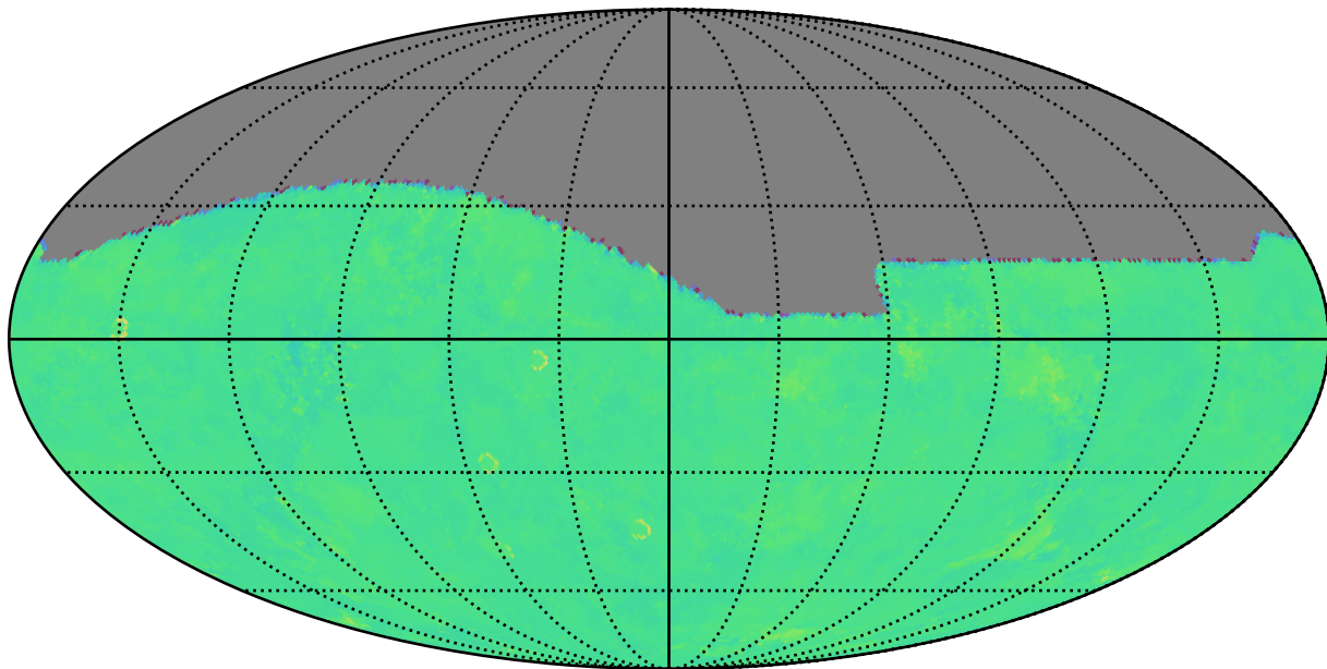
ddf_acor_sf10_lsf30_lsr20_v3.4_10yrs g: Kuiper rotTelPos
