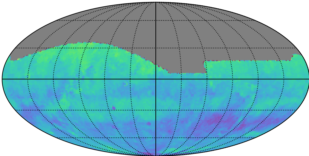
ddf_acor_sf10_lsf30_lsr20_v3.4_10yrs i: Kuiper rotSkyPos
