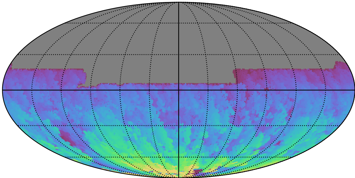
ddf_acor_sf10_lsf30_lsr20_v3.4_10yrs All sky y band: Max HA
