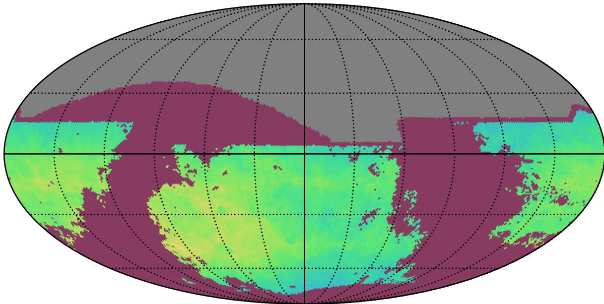
ddf_acor_sf10_lsf30_lsr10_v3.4_10yrs i: NgalScale
