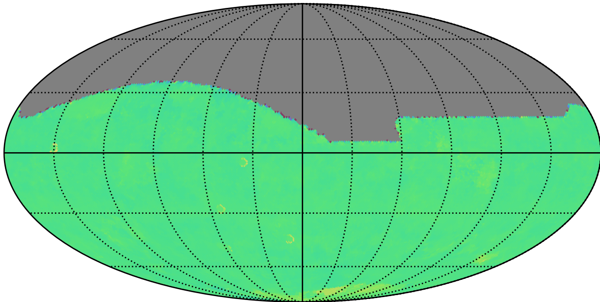
ddf_acor_sf10_lsf30_lsr10_v3.4_10yrs r: Kuiper rotTelPos
