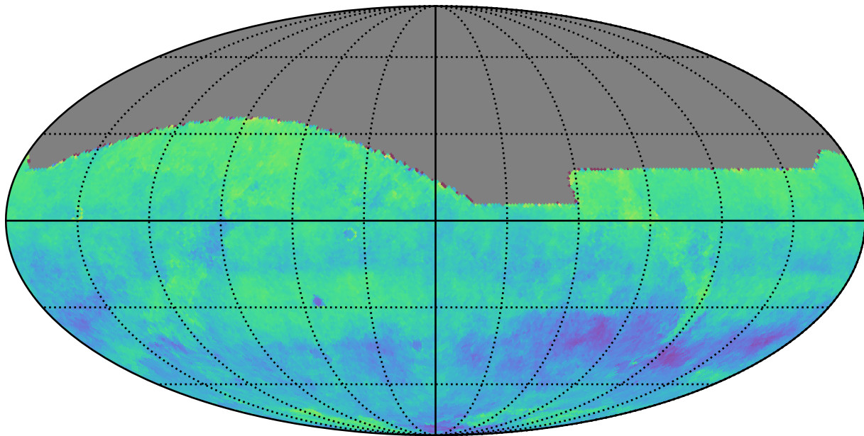
ddf_acor_sf10_lsf30_lsr10_v3.4_10yrs i: Kuiper rotSkyPos
