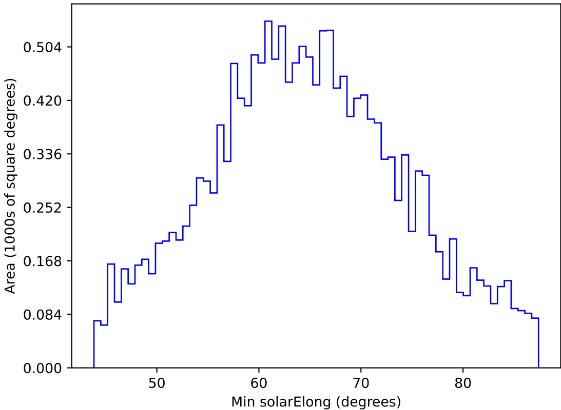
ddf_acor_sf10_lsf30_lsr10_v3.4_10yrs WFD y band: Min solarElong
