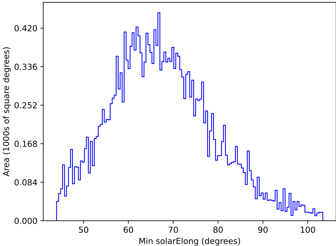
ddf_acor_sf10_lsf30_lsr10_v3.4_10yrs All sky y band: Min solarElong
