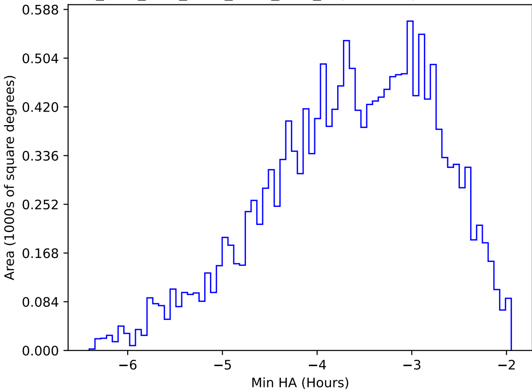
ddf_acor_sf10_lsf30_lsr10_v3.4_10yrs WFD y band: Min HA
