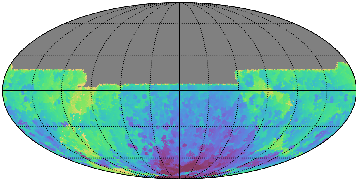
ddf_acor_sf10_lsf30_lsr10_v3.4_10yrs All sky y band: Min HA
