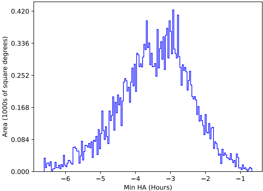
ddf_acor_sf10_lsf30_lsr10_v3.4_10yrs All sky y band: Min HA
