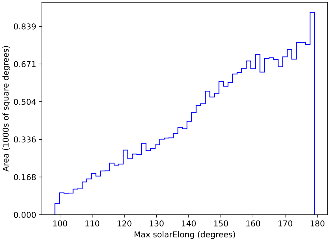
ddf_acor_sf10_lsf30_lsr10_v3.4_10yrs All sky y band: Max solarElong
