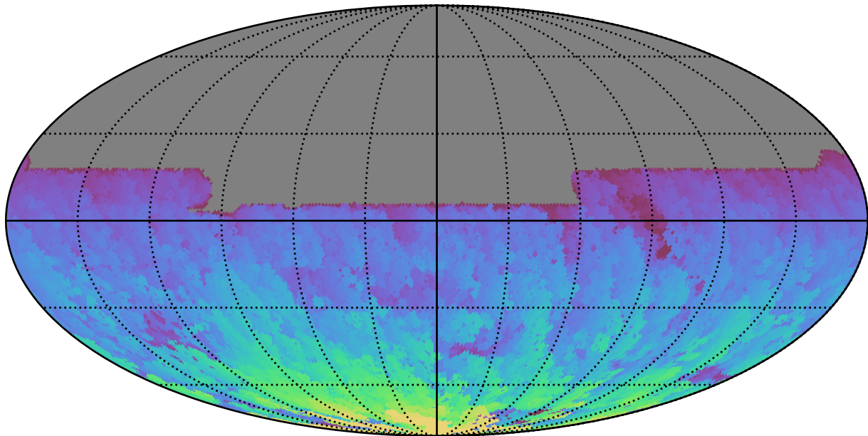
ddf_acor_sf10_lsf30_lsr10_v3.4_10yrs All sky y band: Max HA
