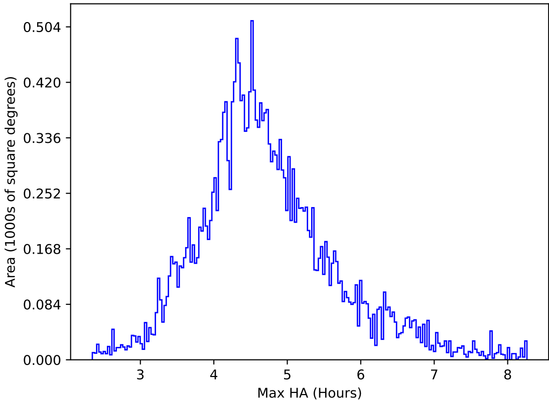
ddf_acor_sf10_lsf30_lsr10_v3.4_10yrs All sky y band: Max HA
