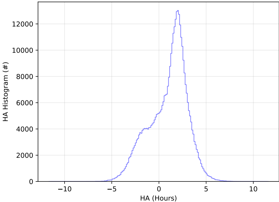
ddf_acor_sf10_lsf30_lsr10_v3.4_10yrs All sky y band: HA Histogram
