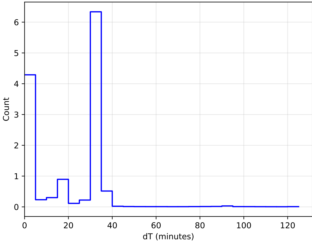
ddf_acor_sf10_lsf30_lsr10_v3.4_10yrs All sky: DeltaT Histogram 1e6
