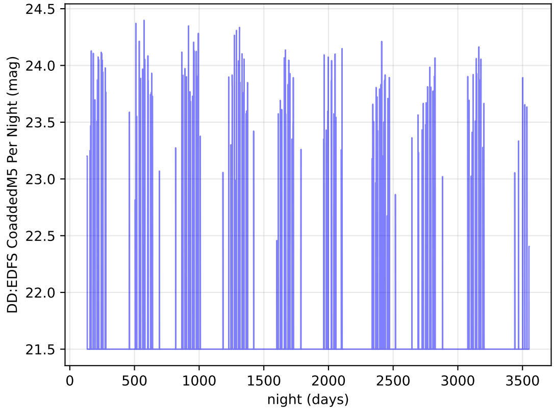
ddf_acor_sf10_lsf30_lsr10_v3.4_10yrs y band: DD:EDFS CoaddedM5 Per Night
