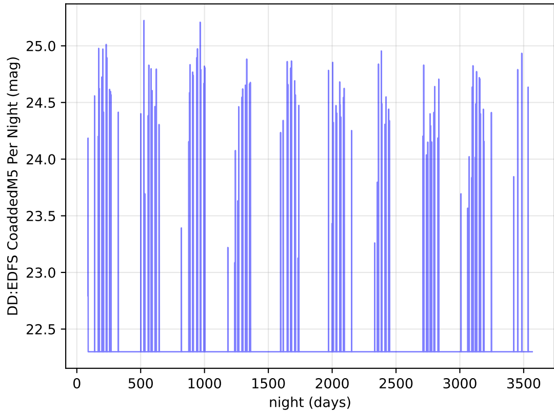
ddf_acor_sf10_lsf30_lsr10_v3.4_10yrs u band: DD:EDFS CoaddedM5 Per Night
