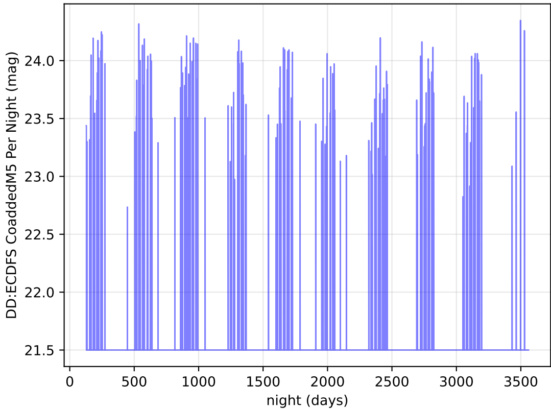
ddf_acor_sf10_lsf30_lsr10_v3.4_10yrs y band: DD:ECDFS CoaddedM5 Per Night
