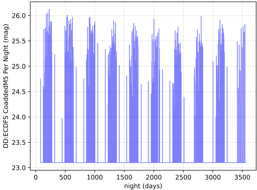
ddf_acor_sf10_lsf30_lsr10_v3.4_10yrs i band: DD:ECDFS CoaddedM5 Per Night
