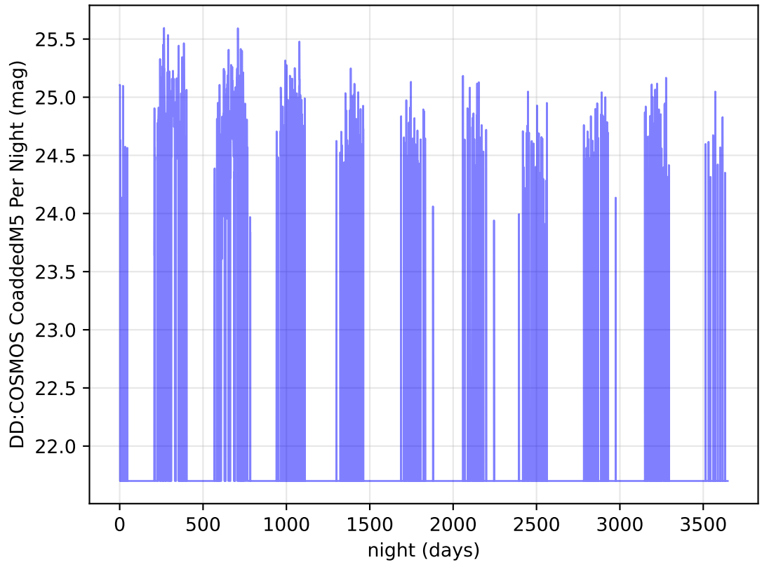
ddf_acor_sf10_lsf30_lsr10_v3.4_10yrs z band: DD:COSMOS CoaddedM5 Per Night
