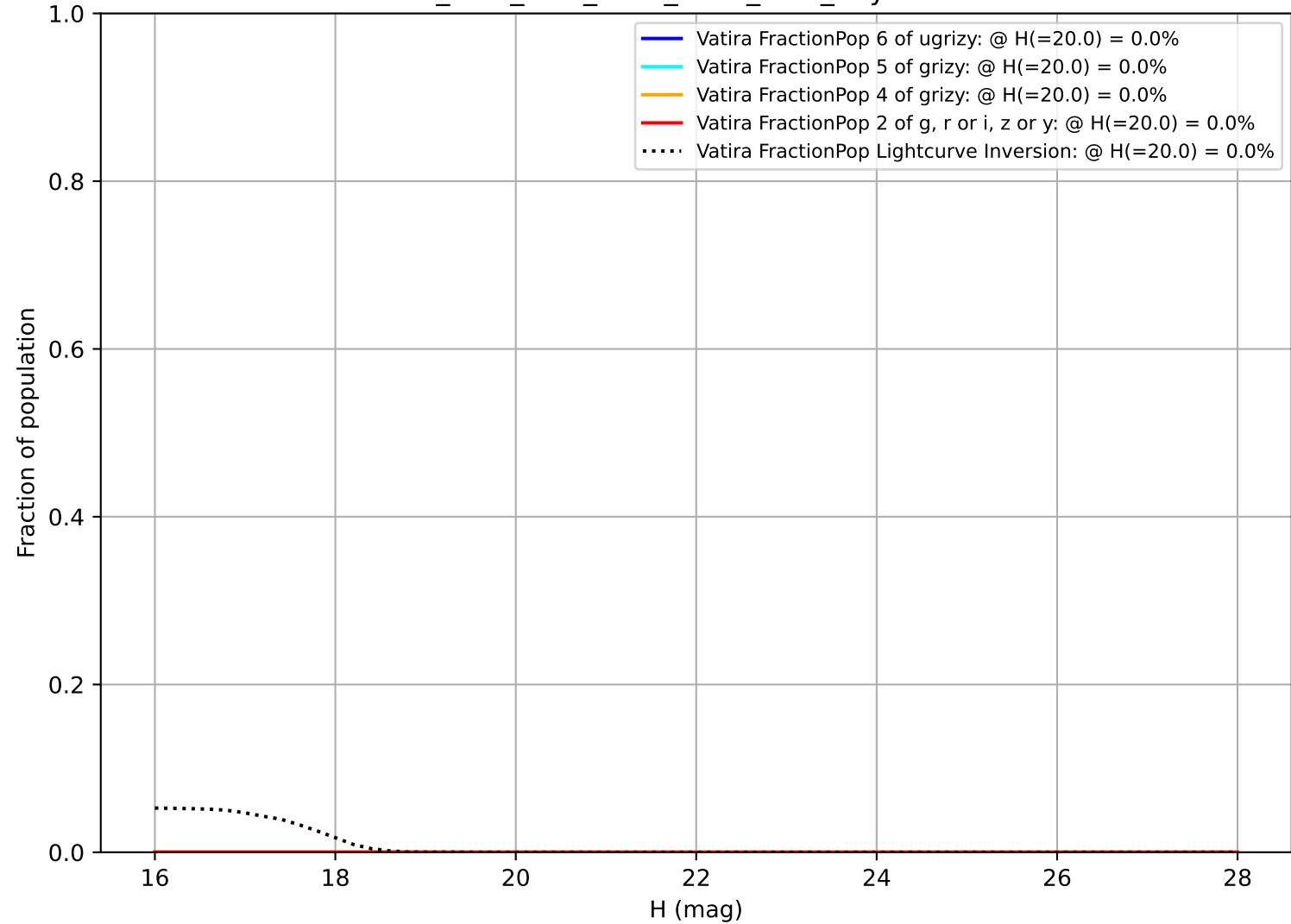
ddf_acor_sf10_lsf20_lsr50_v3.4_10yrs Vatira
