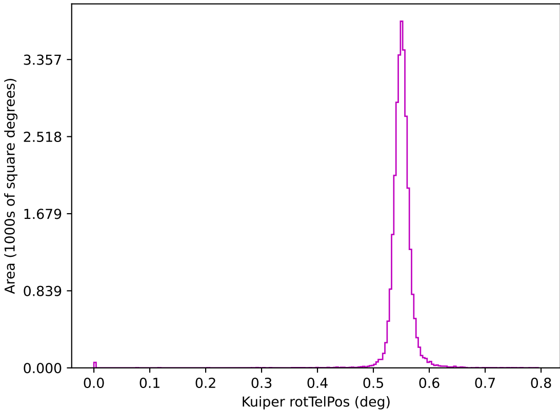
ddf_acor_sf10_lsf20_lsr50_v3.4_10yrs z: Kuiper rotTelPos
