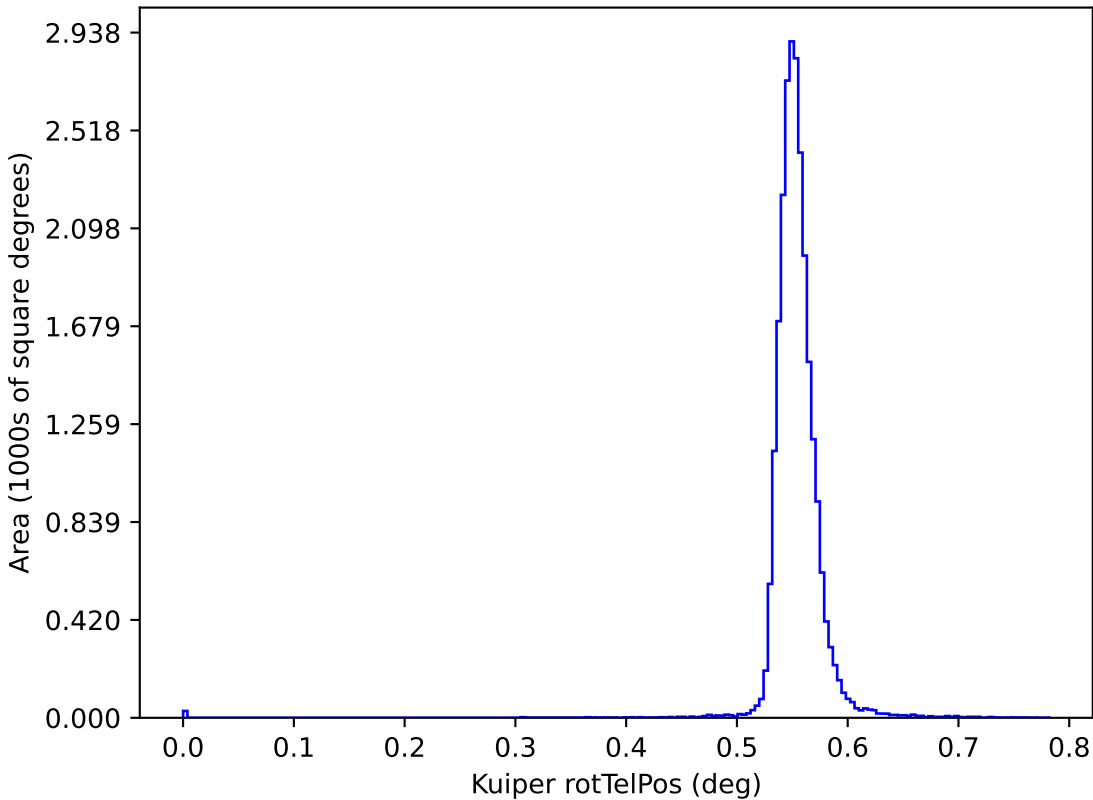
ddf_acor_sf10_lsf20_lsr50_v3.4_10yrs y: Kuiper rotTelPos
