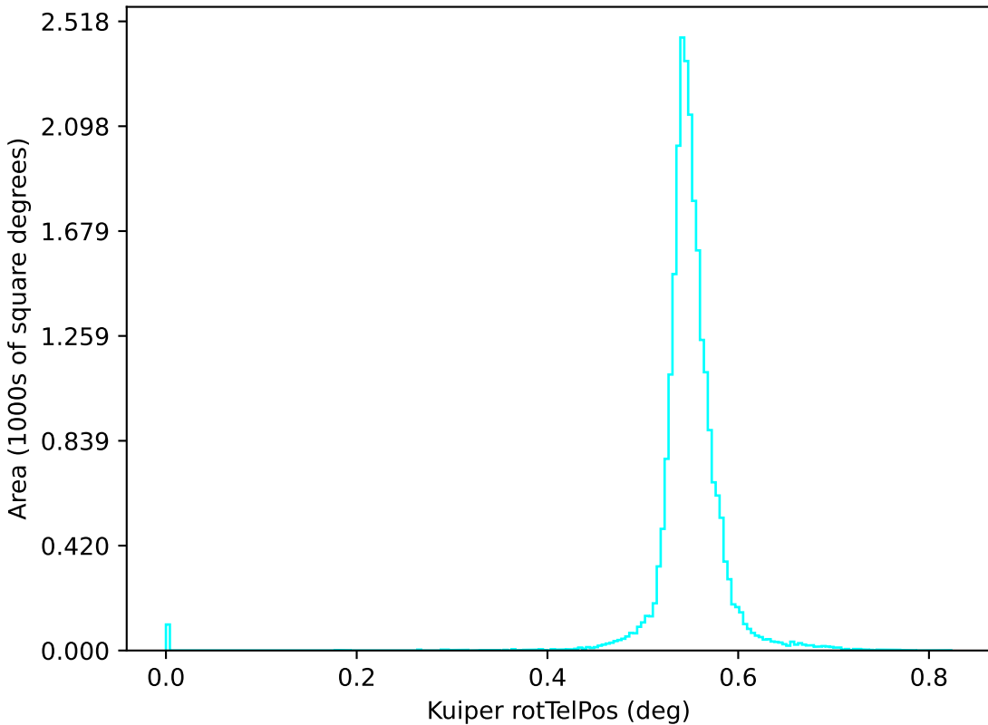
ddf_acor_sf10_ls20_lsr50_v3.4_10yrs u: Kuiper rotTelPos
