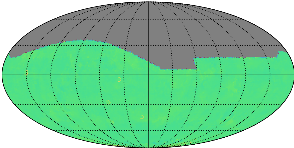
ddf_acor_sf10_lsf20_lsr50_v3.4_10yrs r: Kuiper rotTelPos
