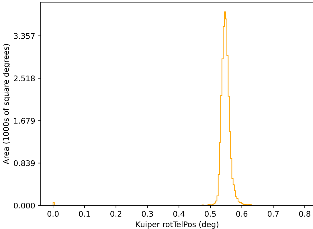
ddf_acor_sf10_lsf20_lsr50_v3.4_10yrs r: Kuiper rotTelPos
