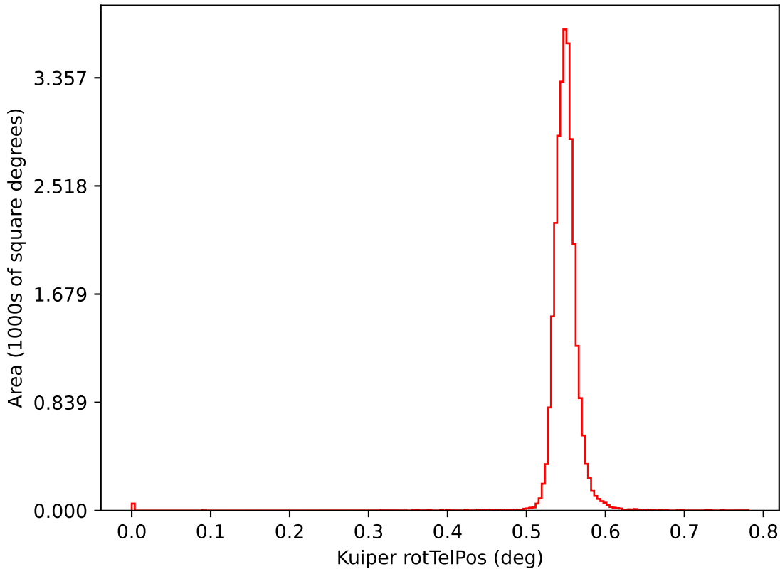
ddf_acor_sf10_lsf20_lsr50_v3.4_10yrs i: Kuiper rotTelPos
