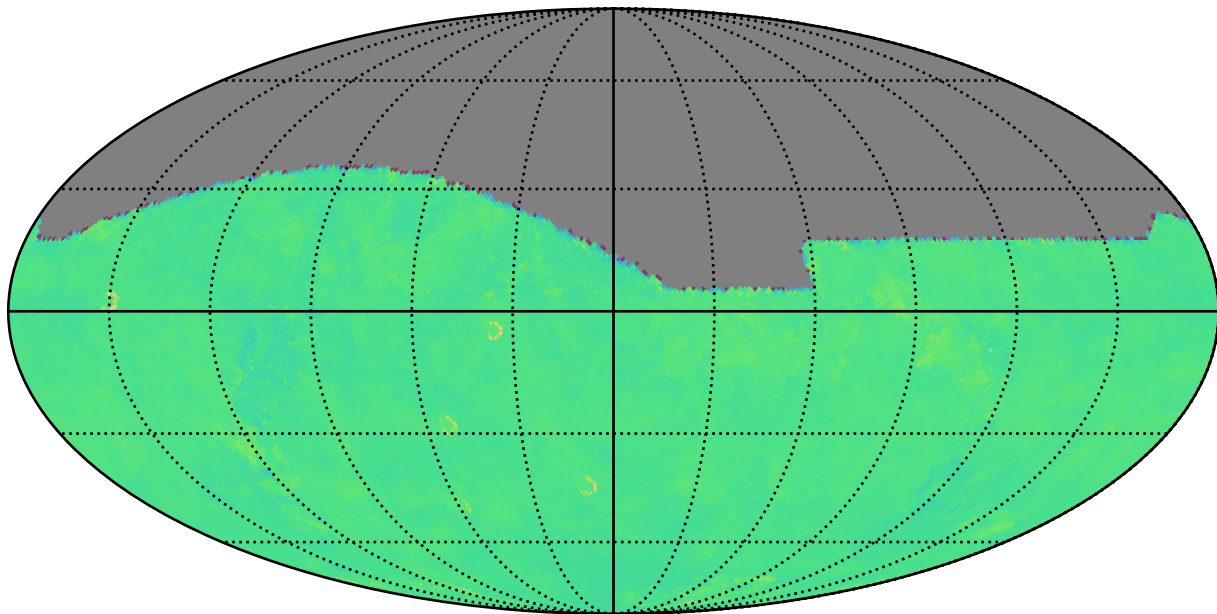
ddf_acor_sf10_lsf20_lsr50_v3.4_10yrs g: Kuiper rotTelPos
