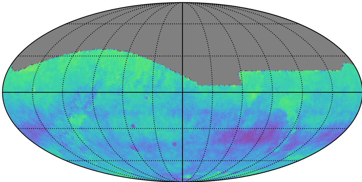
ddf_acor_sf10_lsf20_lsr50_v3.4_10yrs r: Kuiper rotSkyPos
