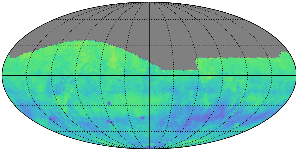
ddf_acor_sf10_lsf20_lsr50_v3.4_10yrs i: Kuiper rotSkyPos
