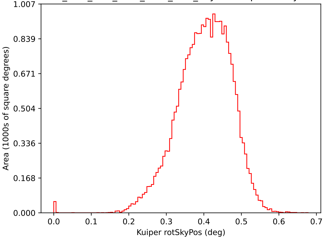
ddf_acor_sf10_lsf20_lsr50_v3.4_10yrs i: Kuiper rotSkyPos
