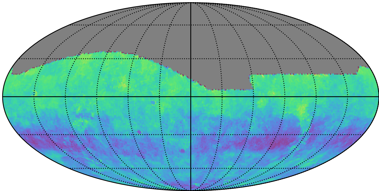
ddf_acor_sf10_lsf20_lsr50_v3.4_10yrs g: Kuiper rotSkyPos
