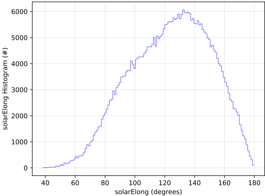
ddf_acor_sf10_lsf20_lsr50_v3.4_10yrs All sky y band: solarElong Histogram
