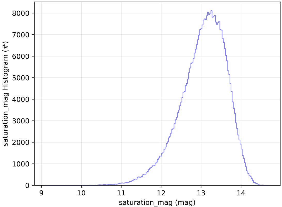
ddf_acor_sf10_lsf20_lsr50_v3.4_10yrs All sky y band: saturation_mag Histogram
