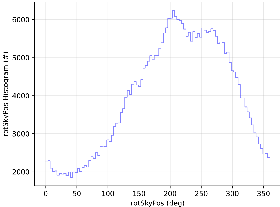
ddf_acor_sf10_lsf20_lsr50_v3.4_10yrs WFD y band: rotSkyPos Histogram
