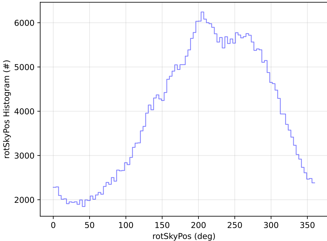
ddf_acor_sf10_lsf20_lsr50_v3.4_10yrs All sky y band: rotSkyPos Histogram
