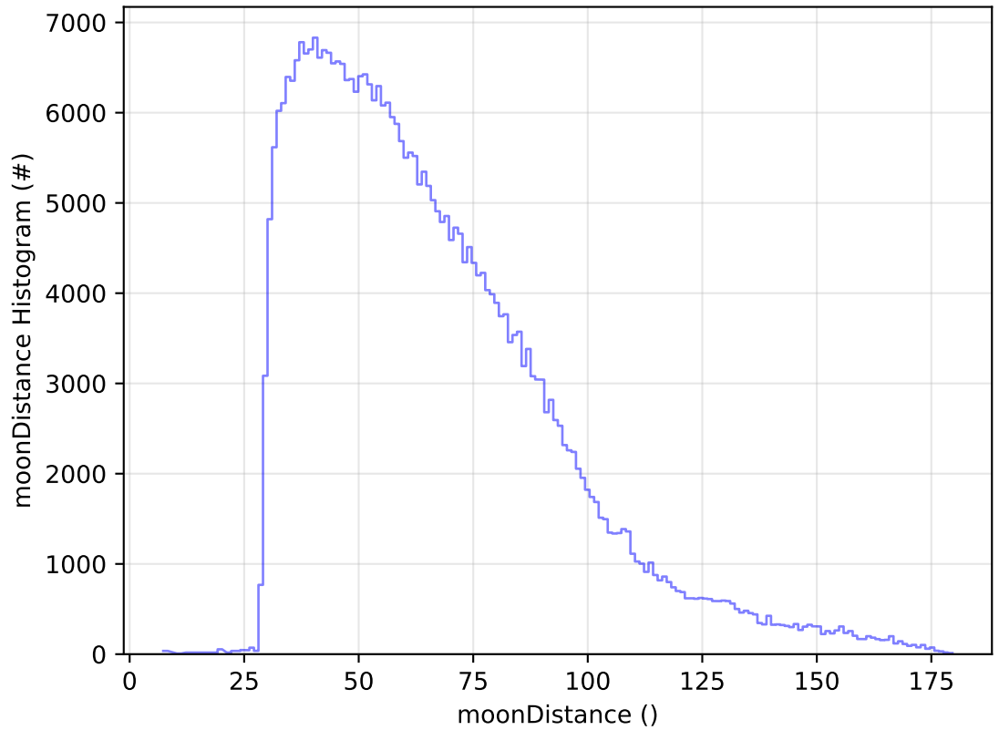
ddf_acor_sf10_lsf20_lsr50_v3.4_10yrs WFD y band: moonDistance Histogram
