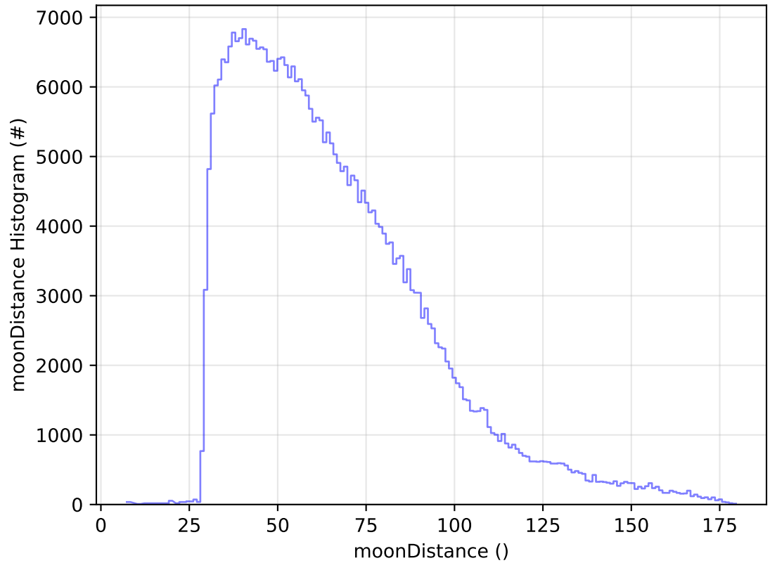
ddf_acor_sf10_lsf20_lsr50_v3.4_10yrs All sky y band: moonDistance Histogram
