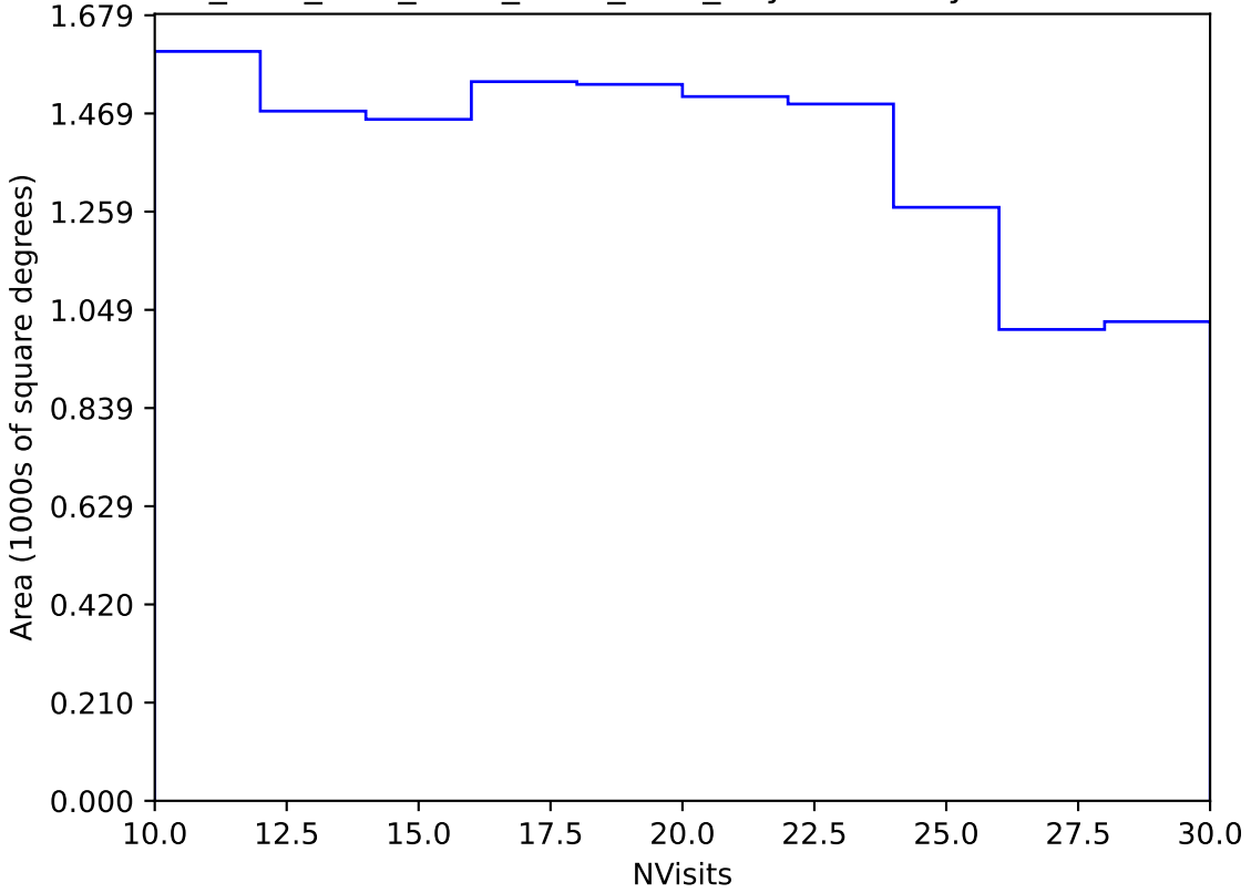
ddf_acor_sf10_lsf20_lsr50_v3.4_10yrs Yr 3-4 y band: NVisits
