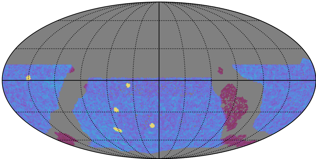
ddf_acor_sf10_lsf20_lsr50_v3.4_10yrs WFD y band: NVisits
