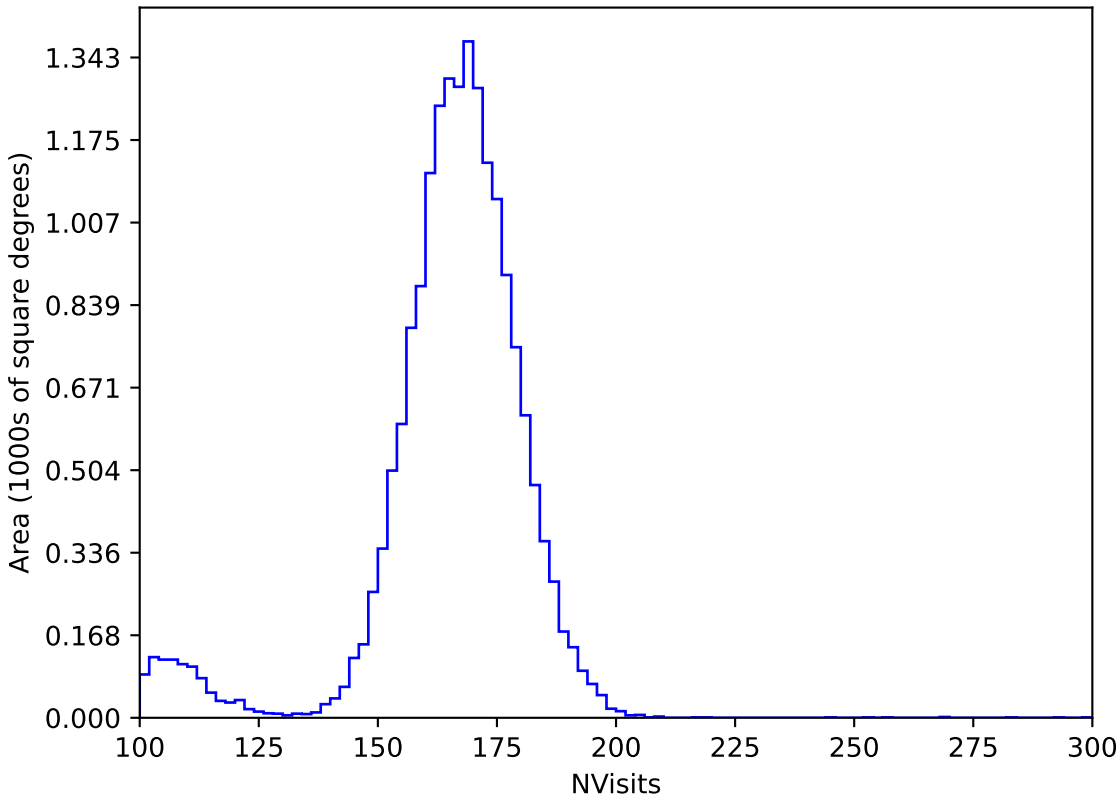
ddf_acor_sf10_lsf20_lsr50_v3.4_10yrs WFD y band: NVisits
