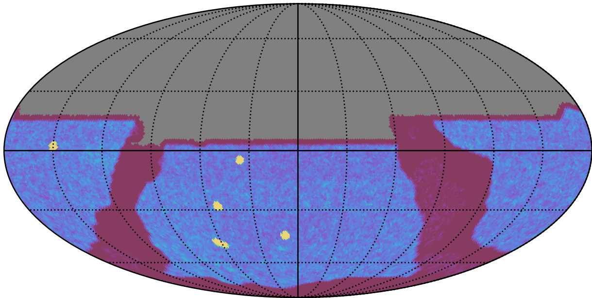
ddf_acor_sf10_lsf20_lsr50_v3.4_10yrs All sky y band: NVisits
