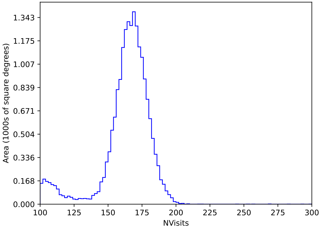
ddf_acor_sf10_lsf20_lsr50_v3.4_10yrs All sky y band: NVisits
