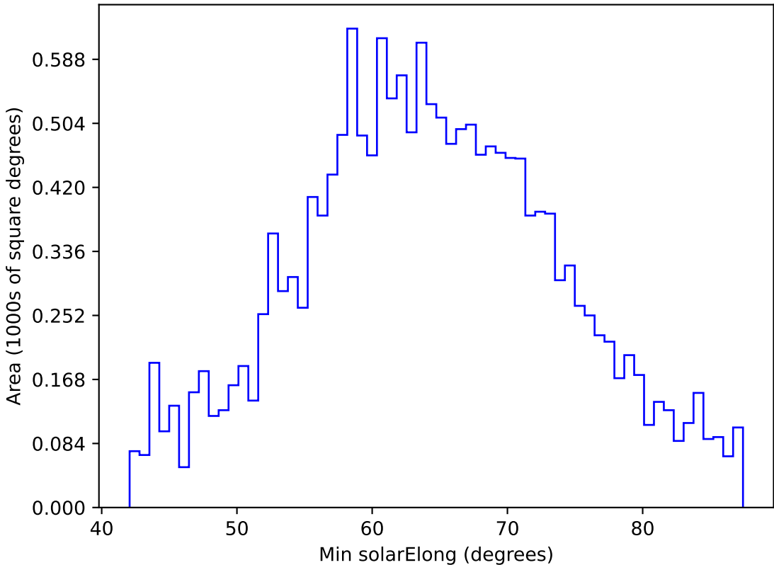
ddf_acor_sf10_lsf20_lsr50_v3.4_10yrs WFD y band: Min solarElong
